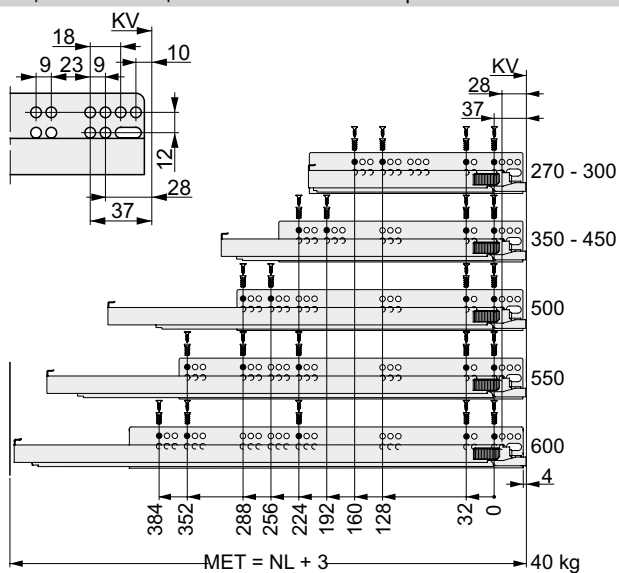
Позиции на захващане за плъзгач с пълно разтягане
