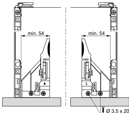
Монтажна позиция за предни щипки
